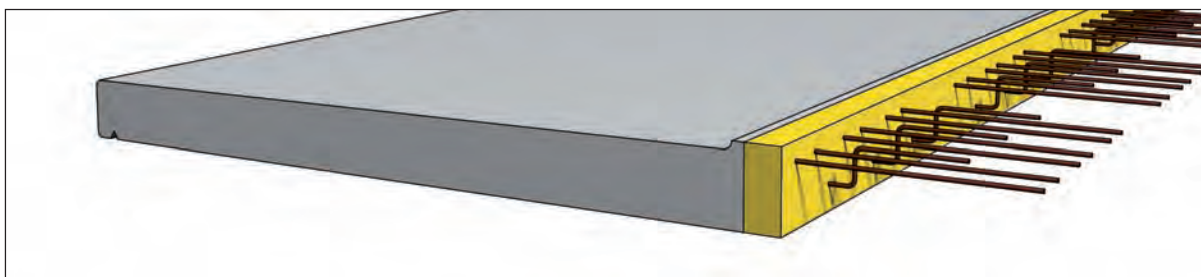
Typ 3. Inspänd med köldbryggebrytande isoleringsmodul
