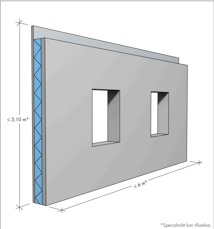
Sektion LK Fasadvägg
