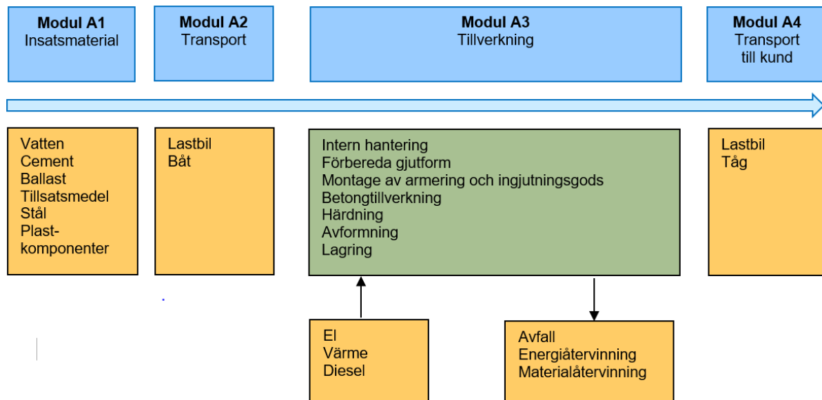
Figur 2 Flödesschema
